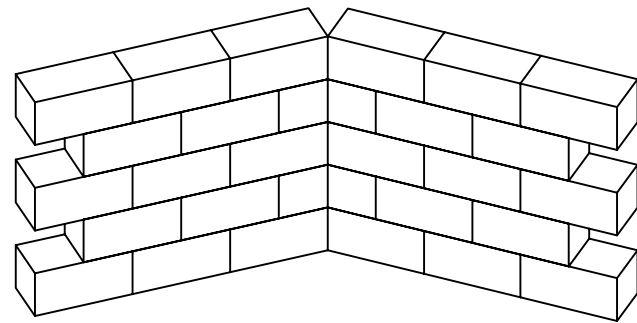
INSIDE ANGLE -NO BATTER (MSE WALL)
