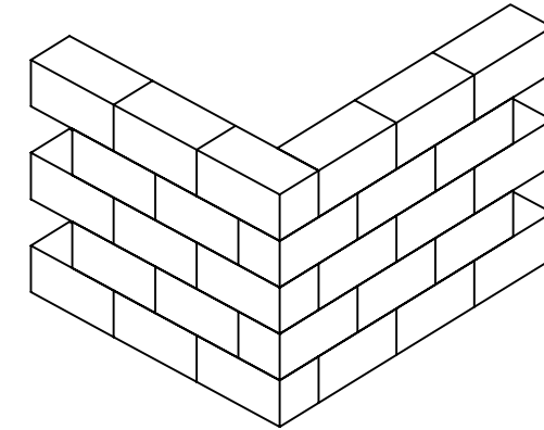
90° CORNER -NO BATTER (MSE WALL)
