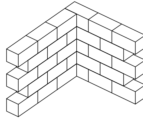
90° CORNER -NO BATTER (MSE WALL)
